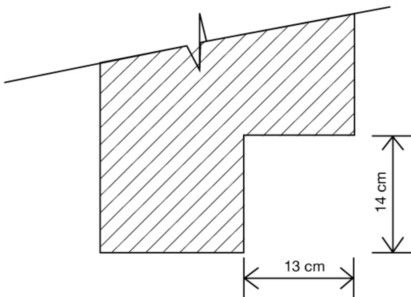
Ventanas hasta 120 cm de altura (sin incluir cajón)
