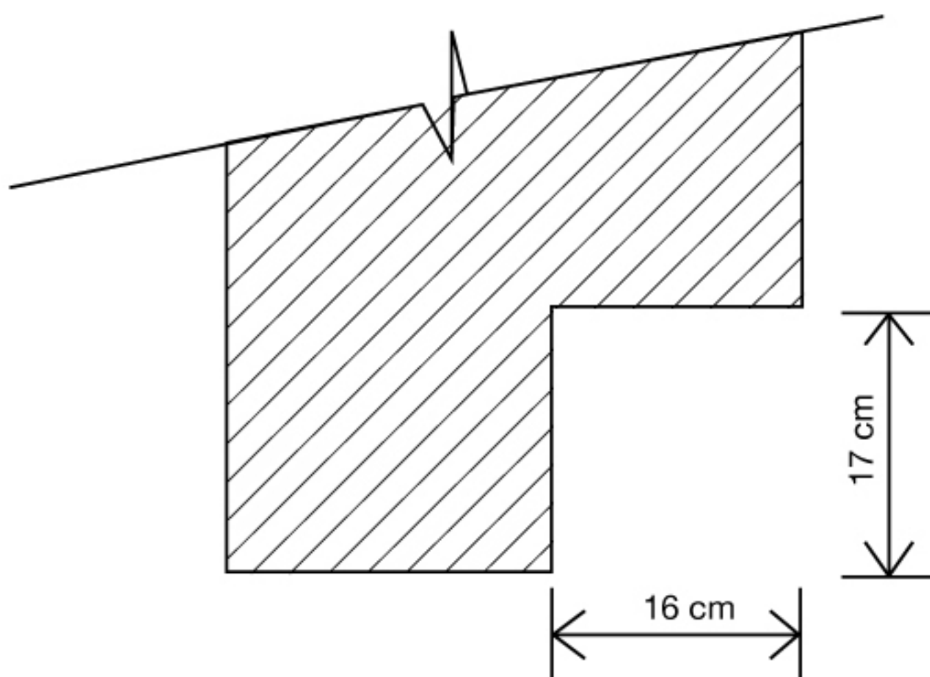
Ventanas y puertas balcón desde 120 cm hasta 210 cm de altura (sin incluir cajón)
